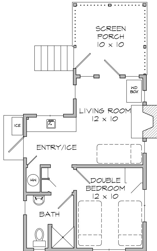
FLOOR PLAN Scale: 1/8" = 1'
