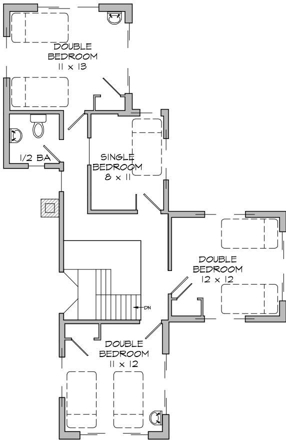
Scale: 3/32" = 1'
